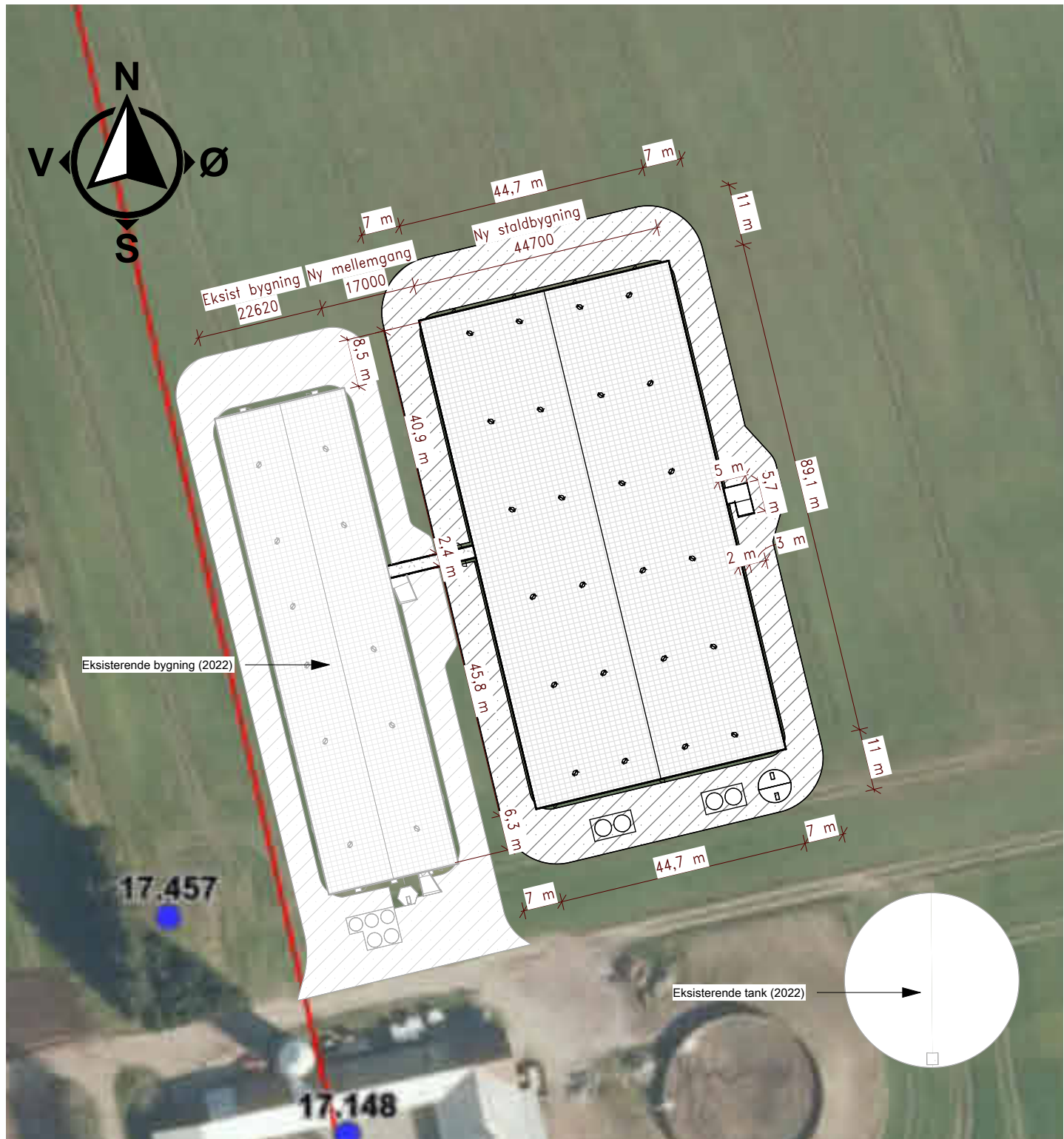
Beliggenhedsplan, 1 : 1000
